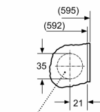
Orificio de la bisagra mín. 12 prof.
